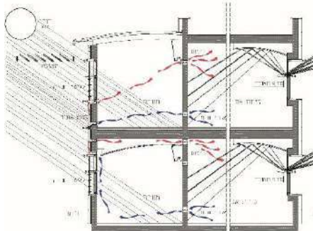
טכניקה אקלימית - חורף קני"מ 1:50
